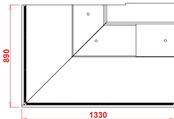
Angle 90° extérieur ECLAIR PA - 23
