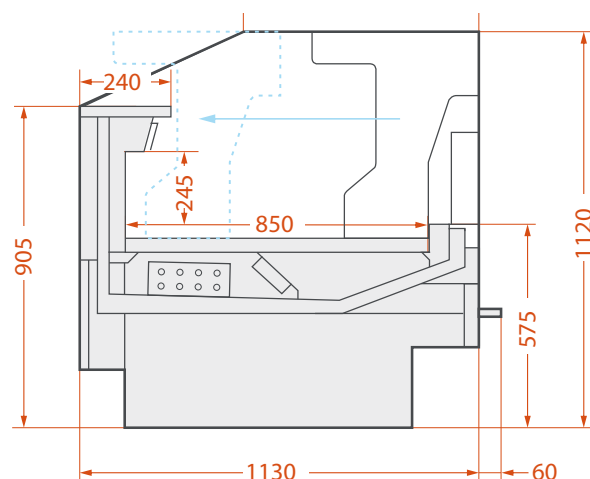
TUCANA VISION - 23 TRANSFORMABLE EN VERSION SELF PAR VITRAGE COULISSANT
