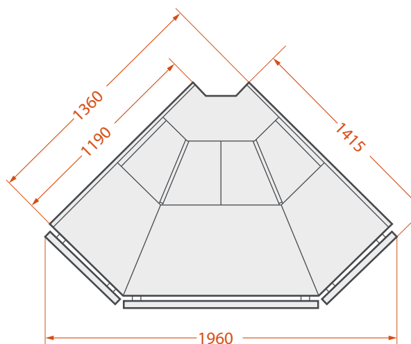
TUCANA VISION ANGLE 90° EXTÉRIEUR
